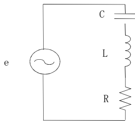
回路図 A
